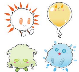
色×元素 ～光る期待のヒミツ～
