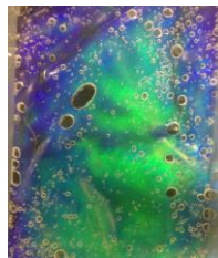
自然界の織りなす神秘的 色彩—構造色
