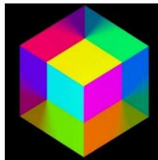
減法混色グラデーション立方体
